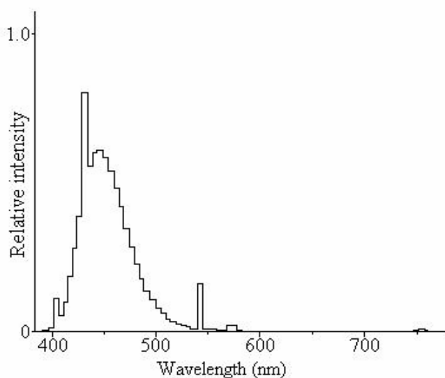
Fig. 2. Spectral characteristics of lamps emitting blue light by Philips (TLD 36W/18) Ryc. 2. Charakterystyka spektralna lamp emitujących światło niebieskie wg firmy Philips (TLD 36W/18)
