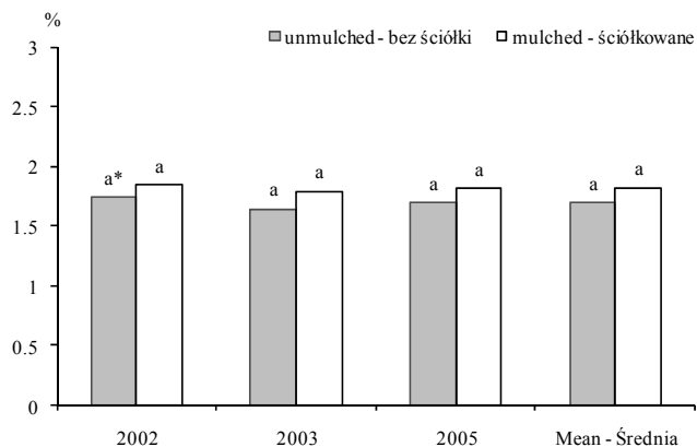
Fig. 3. Effect of black polyethylene mulch on dry matter content in cucumber fruit Ryc. 3. Wpływ ściółkowania gleby czarną folią na zawartość suchej masy w owocach ogórka
