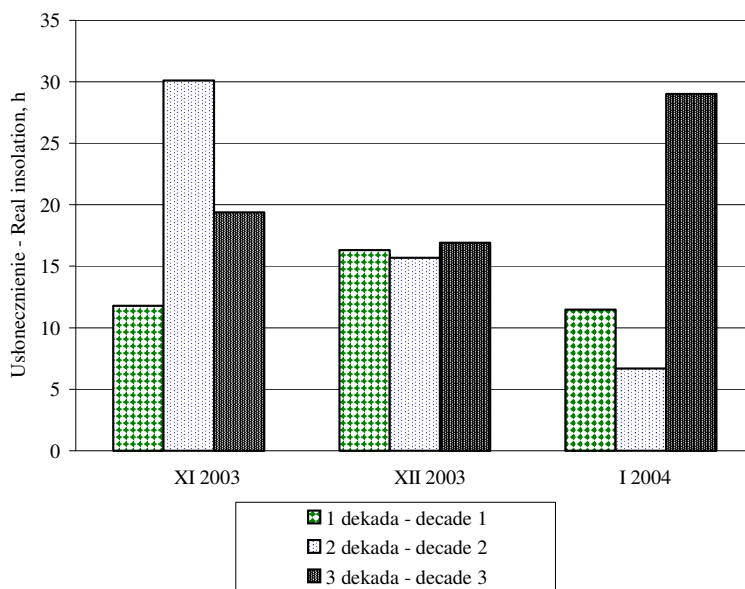
Ryc. 1. Usłonecznienie od listopada 2003 do stycznia 2004 Fig. 1. Real insolation from November 2003 to January 2004
